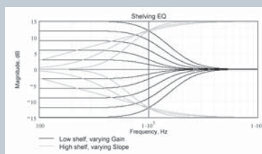
Zwei Shelving Filter (mit PodWare)
