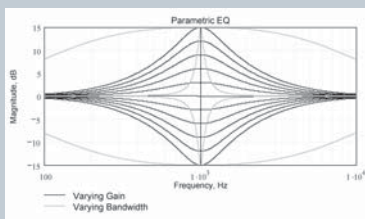
Acht voll-parametrische EQs (mit PodWare)
