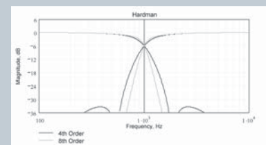
Hardman Filter: Mehr Flankensteilheit bei gleicher Phasenverzerrung für natürliche Klangwiedergabe
